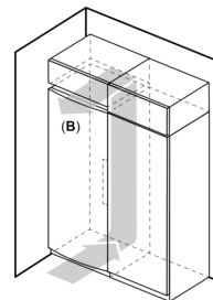
B: Öhu väljalaskeava \geq 200 \text{ cm}^2
