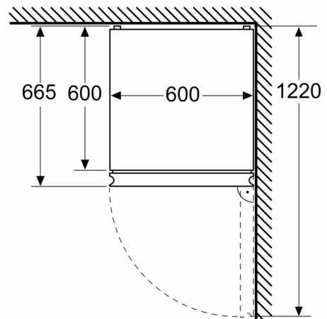
Mõõdud (mm)
