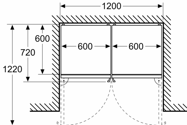
Mõõdud (mm)
