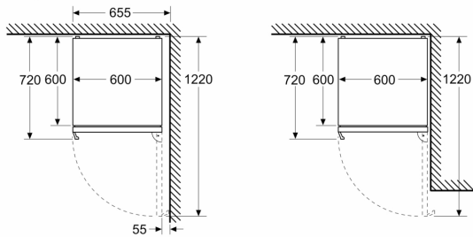
Mõõdud (mm)
