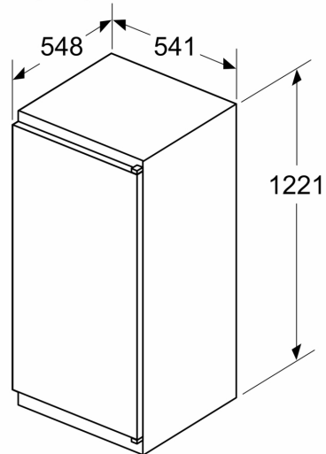
Mõõdud (mm)
