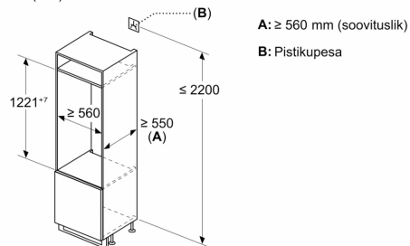
Mõõdud (mm)
