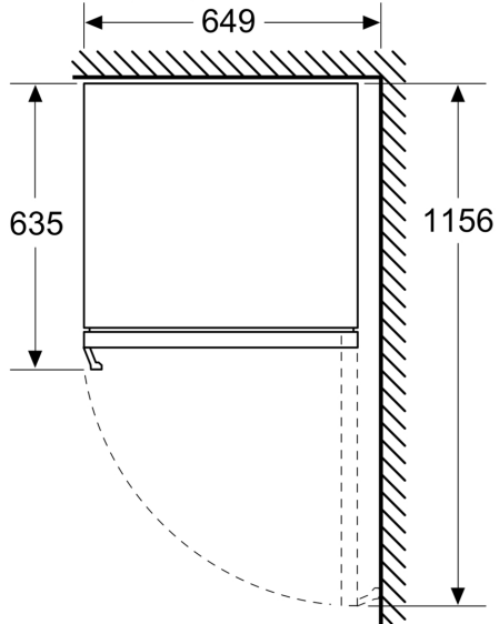
mõõdud (mm)
