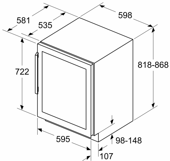
Mõõdud (mm)
