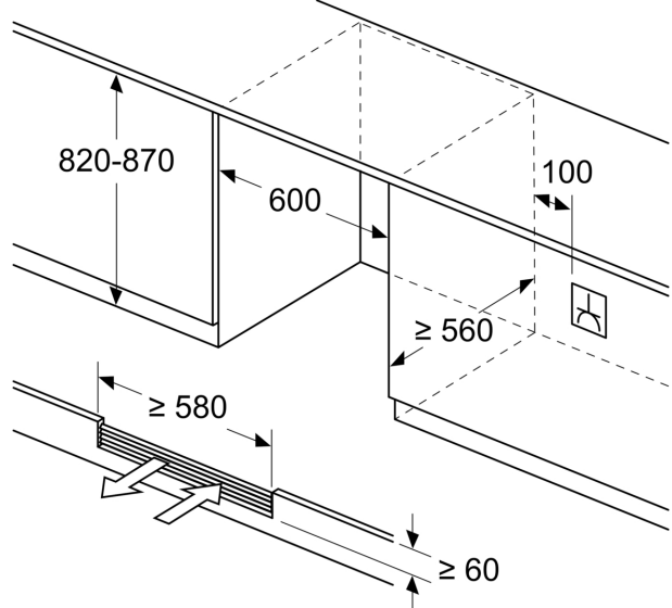
mõõdud (mm)
